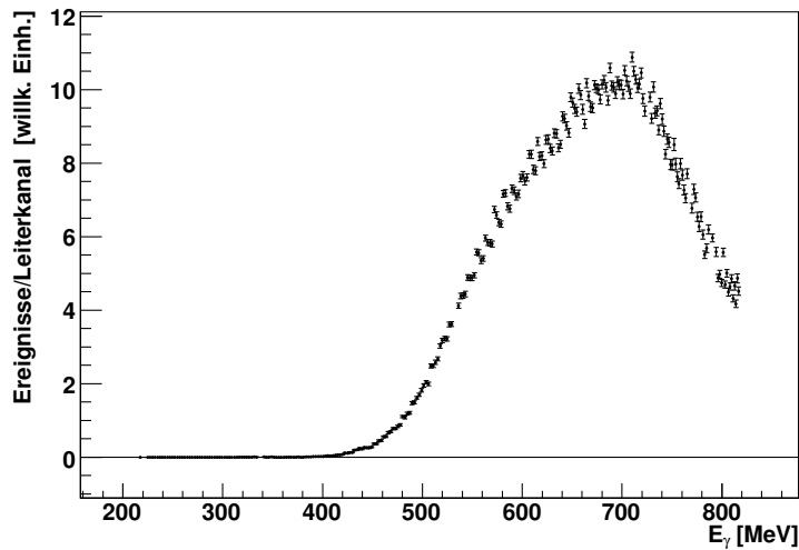
Anregungsfunktion fuer p \pi^+ \pi^- (in exp. Akzeptanz)
