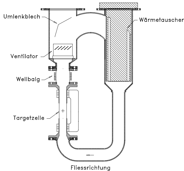
Abb. 4.4: Aufbau des Targetkreislaufs: Das verflüssigte Targetmaterial wird durch die Zelle gepumpt, wo es durch den Strahl aufgeheizt wird, und dann im Wärmetauscher wieder abgekühlt. (Bild nach [23])
