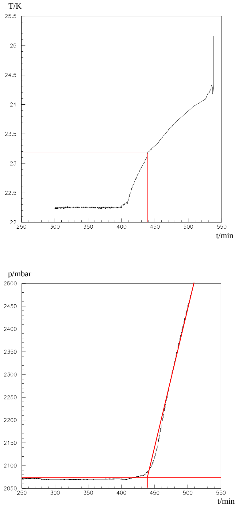
Abb. 5.8: Temperatur- und Druckverlauf im Target während des Aufwärmens im Jahr 2002. Der Druckverlauf vor und nach Erreichen des Siedepunkts wird durch zwei Geraden angenähert.
