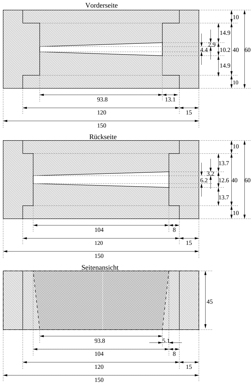
Abb. A.3: Maße des 1.8-msr-Kollimators
