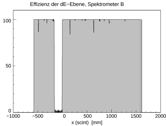
Abb. 5.12: Test der Szintillatoreffizienz am Beispiel der dE-Ebene von Spektrometer B, mit ausgeschaltetem vierten Streifen. Dargestellt ist die Anzahl der in der dE-Ebene registrierten Ereignisse entlang der Längsachse des Spektrometers, normiert mit allen Ereignissen, für die die Driftkammern eine Spur berechnen konnten und für die die ToF-Ebene angesprochen hat. Die Stellen, bei denen das Ergebnis von 100% abweicht, liegen bei den Koordinaten der Stoßstellen beider Ebenen.
