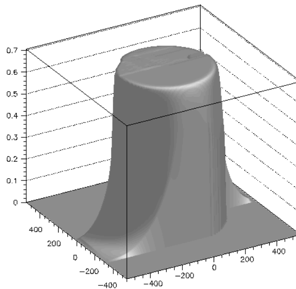
Abb. 3.3: Feldkarte des Short-Orbit-Spektrometers bei einem Feld von 0.7 Tesla, zusammengesetzt aus zwei Einzelmessungen (erkennbar an der Lücke in der Mitte). x- und y-Achse sind in mm, wobei der Ursprung in der Mitte des Polschuhs liegt.
