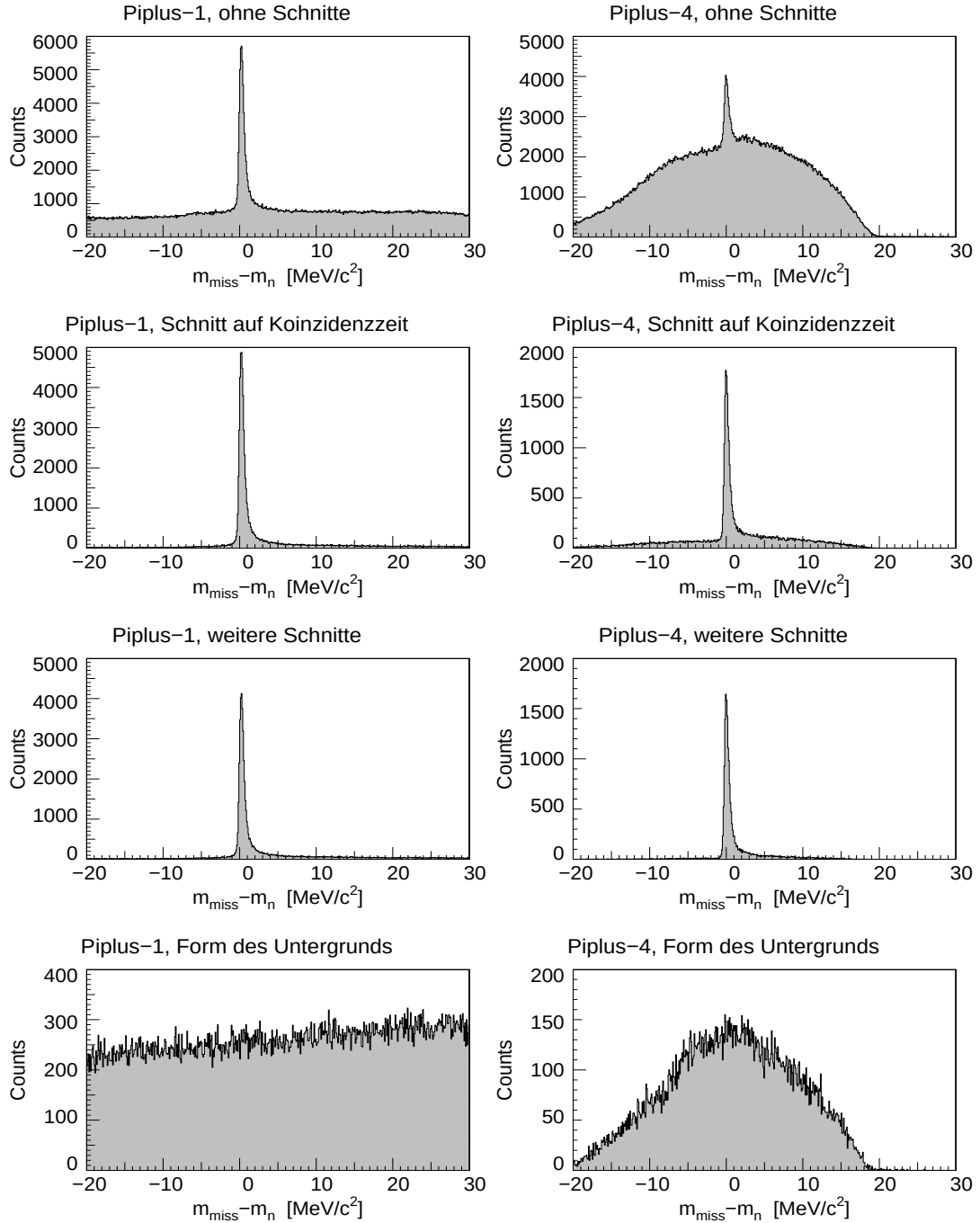
Abb. 5.7: Spektren der fehlenden Masse für die Kinematiken Piplus-1 (links) und Piplus-4 (rechts) (Messung 2000). Gezeigt ist die Reduzierung des Untergrunds durch Schnitt auf den Koinzidenzzeitpik und durch Schnitt auf Impulsakzeptanz, y -Koordinate an der Eintrittsstütze ( y_T ) und Čerenkov-Veto. In der untersten Zeile ist der Untergrund gezeigt, der sich ergibt, wenn auf Ereignisse außerhalb des Koinzidenzzeitpiks geschnitten wird, die alle anderen Schnitte erfüllen. Es handelt sich dabei also nicht um die Ereignisse, die zwischen den Spektren der ersten Zeile und denen der dritten Zeile verworfen wurden. Die Bedeutung der einzelnen Schnitte und des Untergrunds wird in Kapitel 5.3 erklärt.
