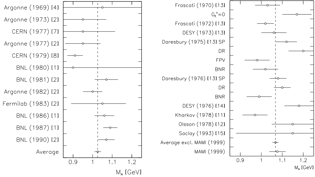
Abb. 1.1: Zusammenstellung der Welt Daten für die axiale Masse, links aus Neutrinostreuung, rechts aus Elektropionproduktion (aus [2]).
