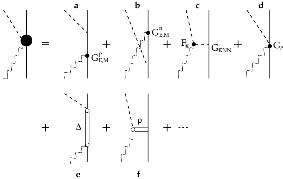
Abb. 2.3: Aufspaltung der Produktionsamplitude für geladene Pionen in nicht-resonante Born-Terme ( a bis d ) und resonante Terme (ab e ):
