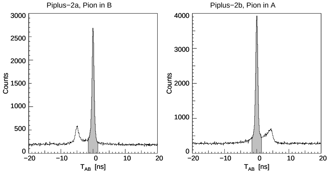
Abb. 5.4: Auf Bahnlängeneffekte korrigierter und ansonsten ungeschnittener Koinzidenzzeitpik für die Kinematiken Pionus-2a (links) und Pionus-2b (rechts) (Messung 2000); der grau markierte Bereich wird akzeptiert
