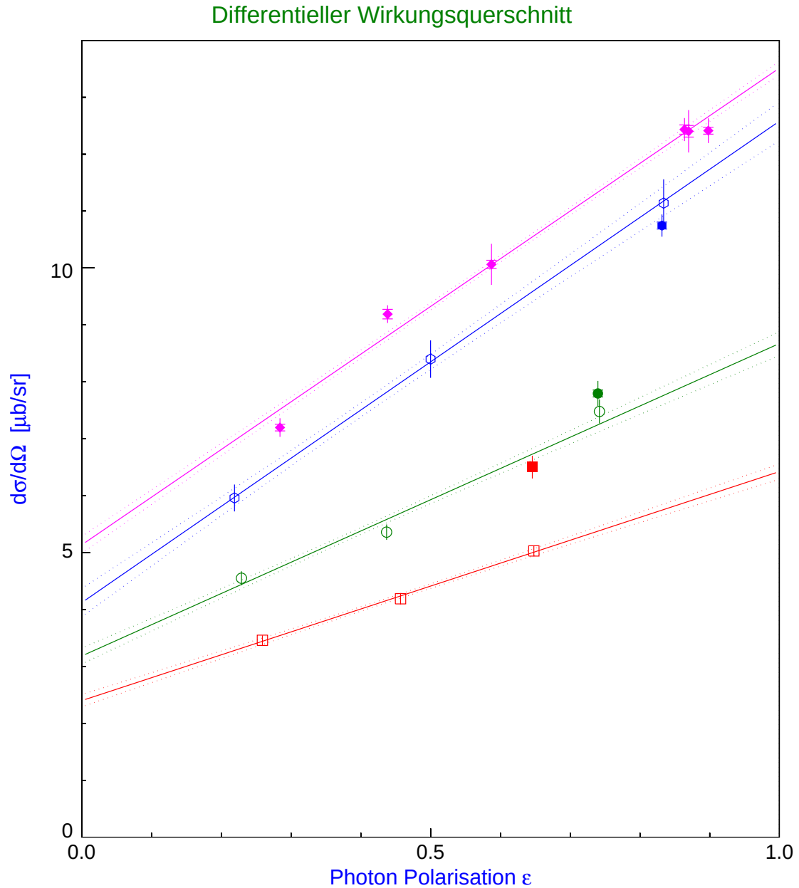
Abb. 6.1: Ergebnisse der Messungen 2000 im Vergleich mit den bisherigen Messungen. Die einzelnen Messungen sind folgendermaßen gekennzeichnet:
