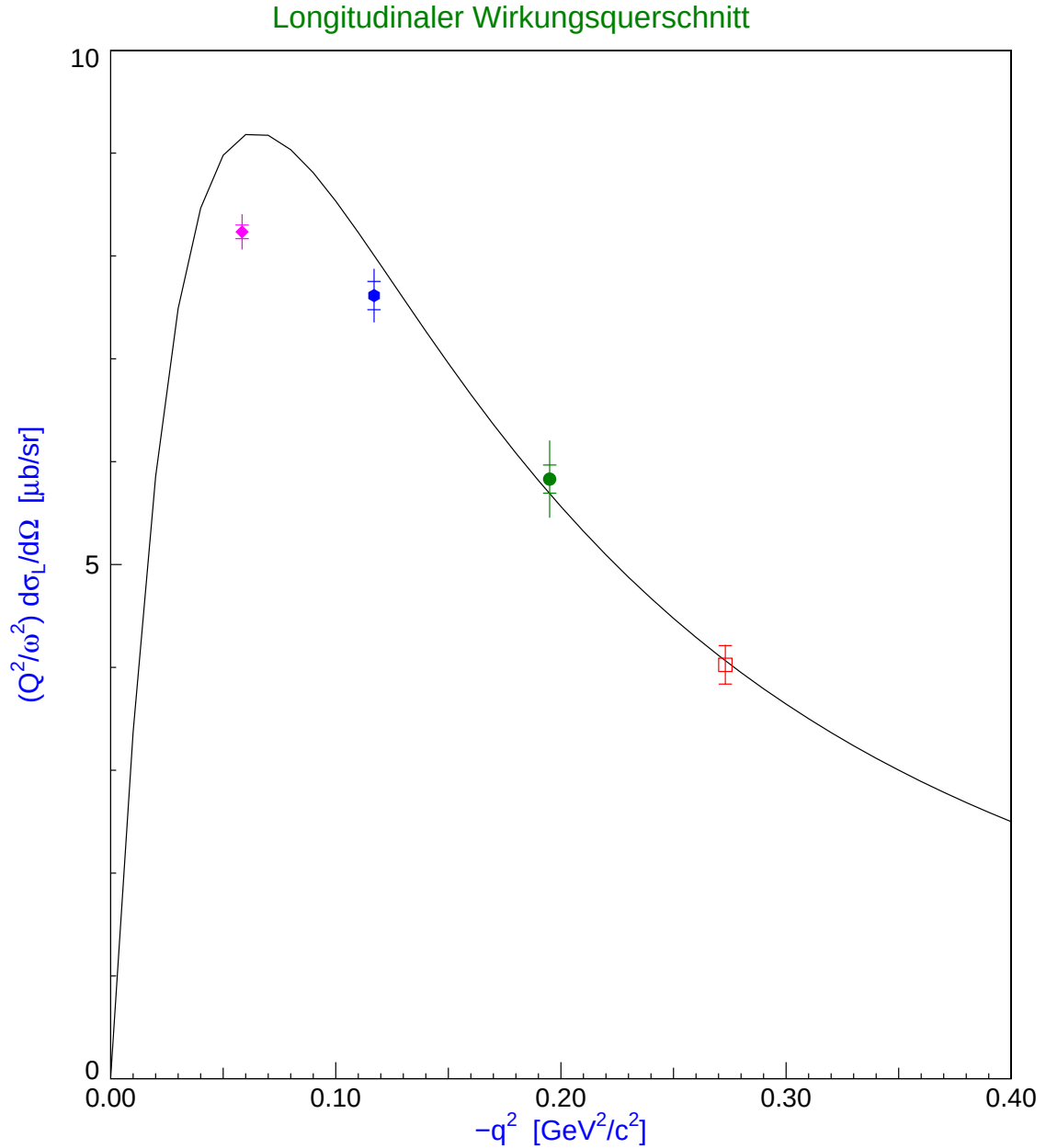
Abb. 6.5: Ergebnisse für den longitudinalen Anteil des Wirkungsquerschnitts der Messungen 2000 und 2002. Eingezeichnet sind die neuen Werte für Q^2 = 0.058, 0.117 und Q^2 = 0.195 ( \text{GeV}/c ) 2 , der Wert für Q^2 = 0.273 ( \text{GeV}/c ) 2 stammt aus [3], ebenso die eingezeichneten Kurven, die an die alten Daten angepaßt wurden. Bei den neuen Werten markieren die Fehlerbalken den Gesamtfehler und die Unterteilung der Balken die Größe des statistischen Anteils.
