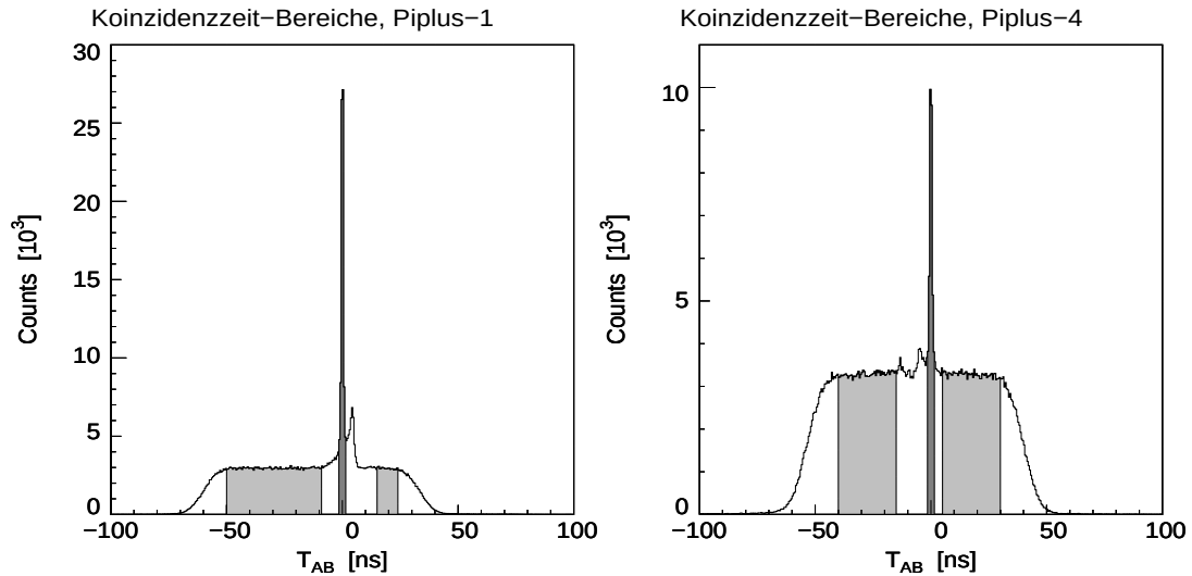
Abb. 5.6: Koinzidenzzeitbereiche für die Kinematiken Piplus-1 und Piplus-4 (Messung 2000); der dunkelgrau markierte Bereich wird akzeptiert, der hellgrau markierte dient zur Bestimmung des Untergrunds
