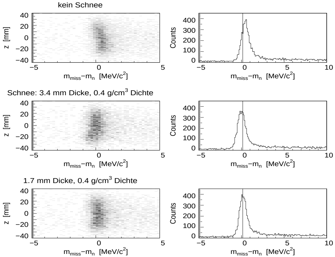
Abb. 5.9: Fehlende Masse für verschiedene in der Analyse angenommene Parameter Schneedicke und -dichte, Kinematik Piplus11 (Messung 2002). Gezeigt sind jeweils die Verteilung der fehlenden Masse gegen die Längsachsenkoordinate und der sich ergebende Pik. Ohne Schnee (oben) ist die Energieverlustkorrektur zu klein, bei zuviel Schnee (mitte) wird überkorrigiert; unten die in der Analyse verwendete Schneedicke. Rechts ist eine Linie bei 0.2 \text{ MeV}/c^2 eingezeichnet, um zu verdeutlichen, daß die Position des Piks für höhere Schneedicke nach links wandert.
