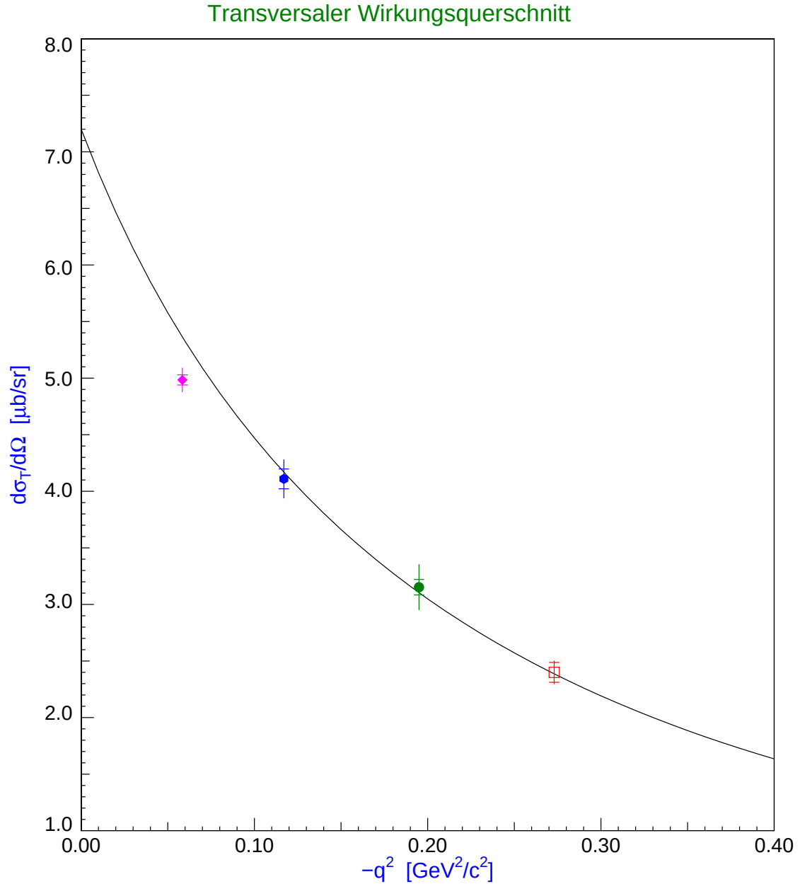
Abb. 6.4: Ergebnisse für den transversalen Anteil des Wirkungsquerschnitts der Messungen 2000 und 2002. Eingetragen sind die neuen Werte für Q^2 = 0.058, 0.117 und Q^2 = 0.195 (GeV/c) 2 , der Wert für Q^2 = 0.273 (GeV/c) 2 stammt aus [3], ebenso die eingezeichneten Kurven, die an die alten Daten angepaßt wurden. Bei den neuen Werten markieren die Fehlerbalken den Gesamtfehler und die Unterteilung der Balken die Größe des statistischen Anteils.
