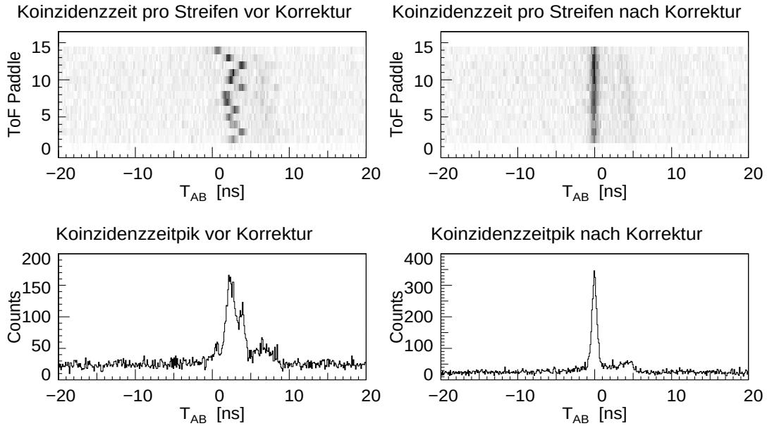
Abb. 5.3: Koinzidenzzeitpik für eine Teilmessung der Kinematik Pionus1 (Messung 2002), links vor, rechts nach der Offsetkorrektur: oben Lage des Piks aufgetragen pro Szintillatorstreifen, unten Gesamtpik aus der Summe der Einzelpiks. Im rechten oberen Spektrum ist rechts vom Hauptpik der vom Myonen verursachte Nebepik zu erkennen, dessen Position im Zeitspektrum vom Szintillatorstreifen, also von der Position in der Fokalebene abhängt.
