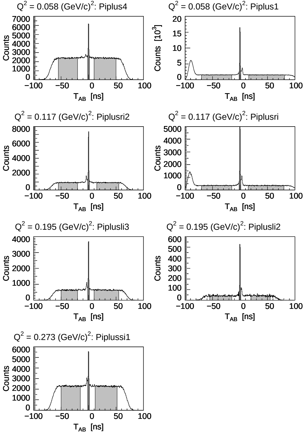
Abb. 5.16: Lage des Untergrundschnitts im Koinzidenzspektrum für einige Kinematiken der 2002-Messung, von oben nach unten nach steigendem Q^2 geordnet. Links Pionnachweis in Spektrometer B, rechts Pionnachweis in Spektrometer A.
