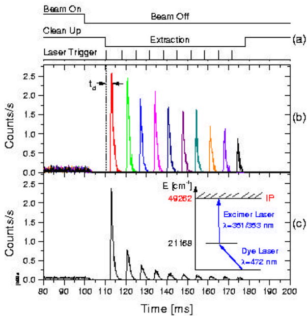
Abb. 2: Zeitlicher Ablauf bei der RIS. Pulsung des Primärstrahls (100 ms an / 100 ms aus), der elektrischen Felder und des Lasers (a). Zeit aufgelöstes Ionensignal ( m=170 u) von 10 einzelnen Laserpulsen (b) und das entsprechende Signal für eine Sequenz von 10 Pulsen (c).
