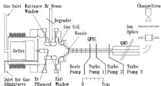
Abb. 1: Aufbau des laserspektroskopischen Experimentes am Emperor Tandem Beschleuniger des MPI für Kernphysik in Heidelberg. Um die Gasverunreinigungen möglichst klein zu halten, ist die optische Zelle in UHV Technik aufgebaut. Das Ar-Gas der Reinheit 6.0 wird durch einen Getter zusätzlich gereinigt. Mit Hilfe eines nat Er-Filamentes kann die Apparatur ohne Strahl getestet und eine Massen- und Wellenlängeneichung durchgeführt werden. Beide Laserstrahlen zur Resonanzionisation wurden über eine einzige Glasfaser zur optischen Zelle transportiert. Der Strahlfleck wurde auf einen Durchmesser von 1,5 cm aufgeweitet und senkrecht zum Er-Strahl eingestrahlt. Der HF-QuadruPol Ion Guide (QPIG) mit einem Innendurchmesser von 3 mm und einem Stabdurchmesser von 3 mm ist in 6 Segmente unterteilt.
