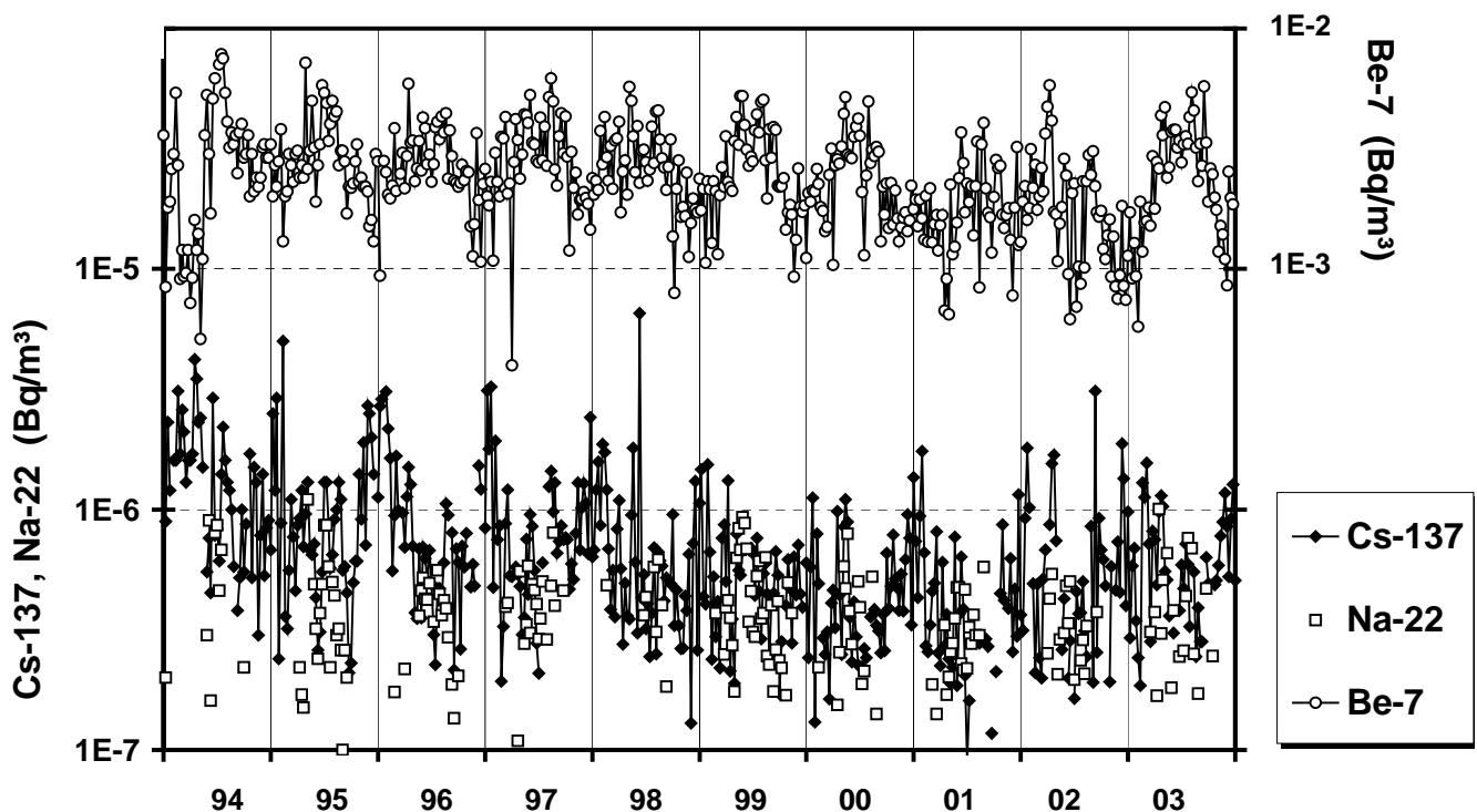
Abb. 1 : Zeitlicher Verlauf der Wochenmittelwerte der Aktivitätskonzentrationen von Cs-137, Be-7 und Na-22 an der Messstation des Instituts für Kernchemie der Johannes Gutenberg-Universität Mainz in den Jahren 1994 bis 2003.
