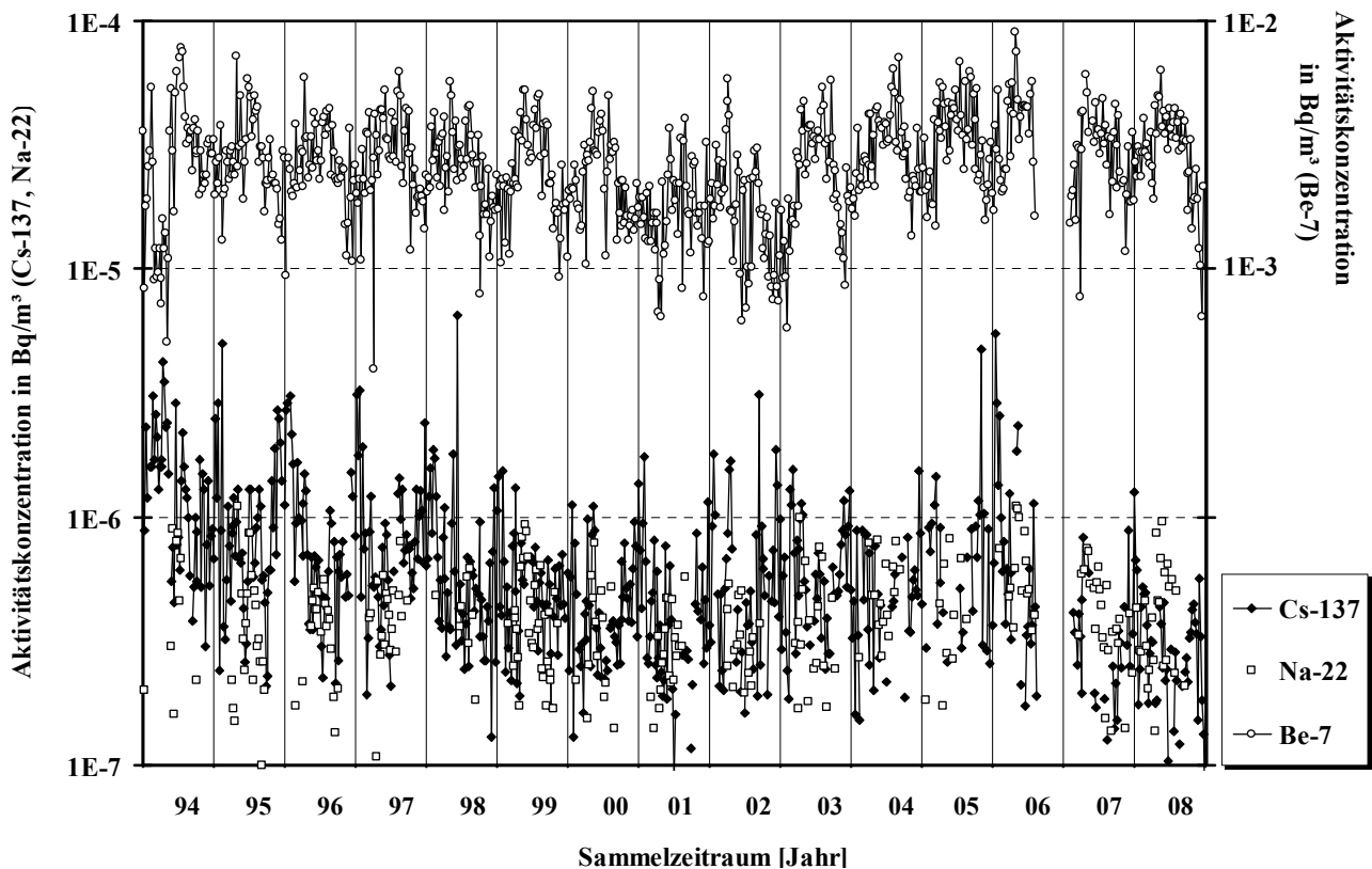
Abb.1 : Zeitlicher Verlauf der Wochenmittelwerte der Aktivitätskonzentrationen von Cs-137, Be-7 und Na-22 an der Messstation des Instituts für Kernchemie der Johannes Gutenberg-Universität Mainz in den Jahren 1994 bis 2008.
